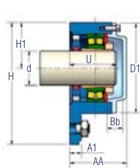
BC - Bloqueada con tapa ciega
