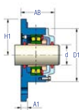
BP -Bloqueada con tapa pasante
