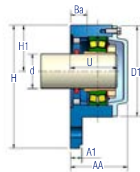
LC - Libre con tapa ciega
