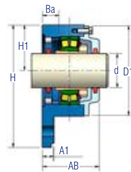
LP - Libre con tapa pasante
