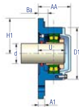
LC - Libre con tapa ciega
