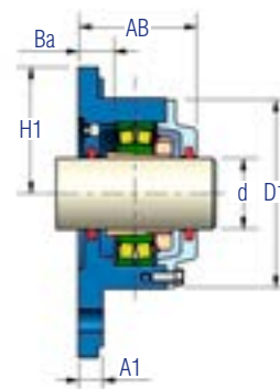
LP -Libre con tapa pasante
